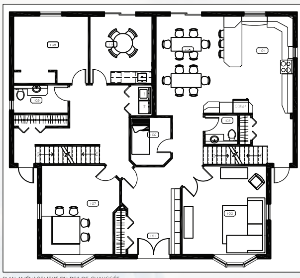
PLAN AMÉNAGEMENT DU REZ-DE-CHAUSSÉE ÉCHELLE: 3/16" = 1'-0"
