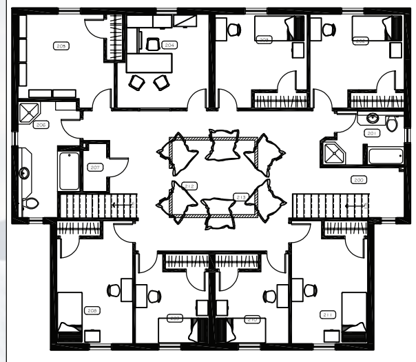
PLAN AMÉNAGEMENT DE L'ÉTAGE ÉCHELLE: 3/16" = 1'-0"
